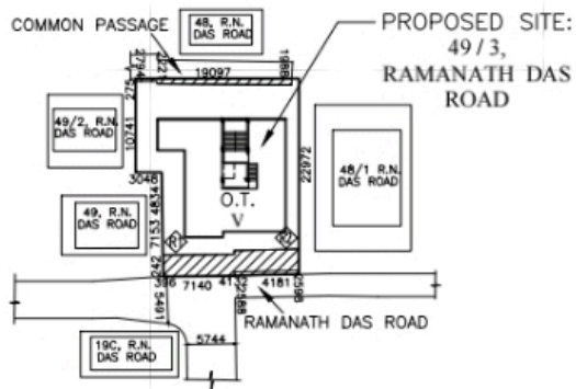
SITE PLAN SCALE-1:600
